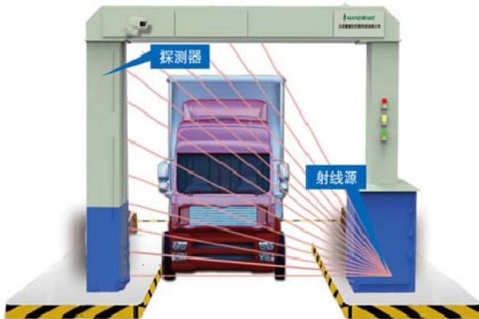
图 9 检查系统工作成像原理
