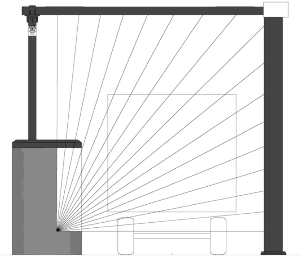
图 14 工作状态的 X 射线线束分布图
