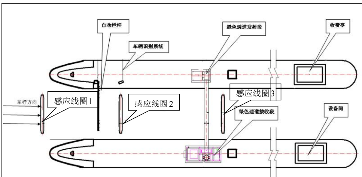
图 13 工作状态演示图
