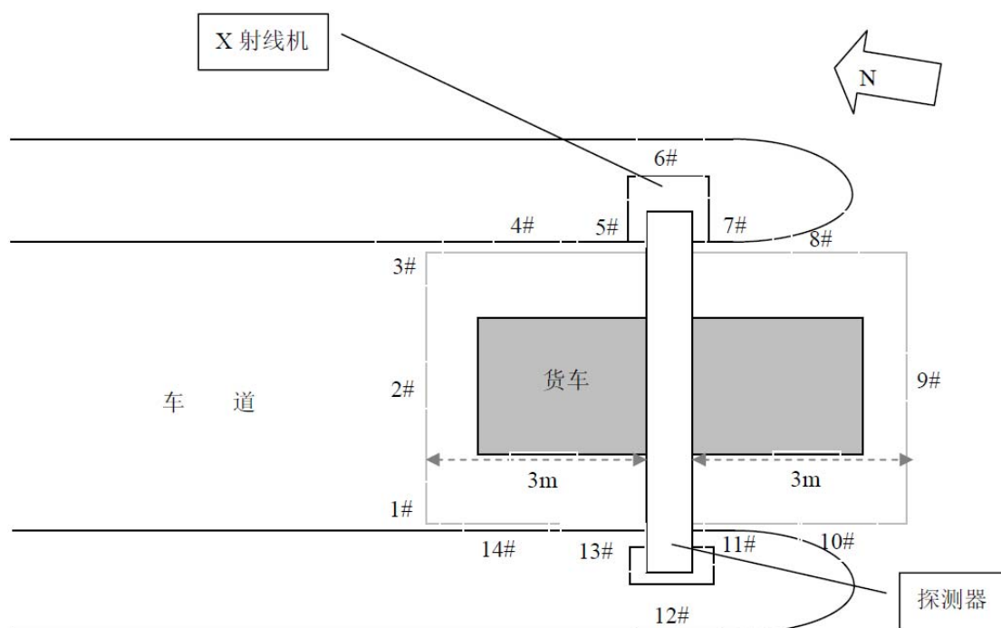
图 15 广东省南雄市韶赣高速梅关收费站绿色通道车辆检查系统 X 射线剂量率检测示意图
