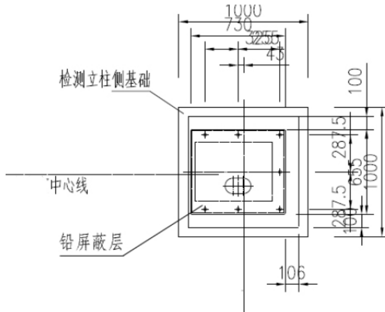
图 11 探测器结构图
